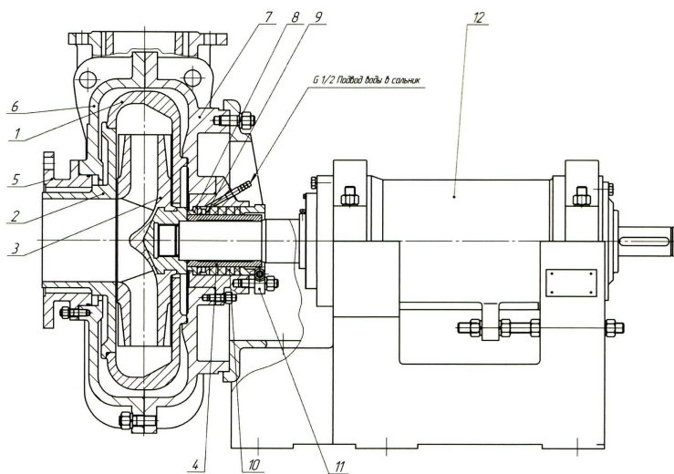
Общий вид грунтовых насосов ГрАТ, ГрАК
