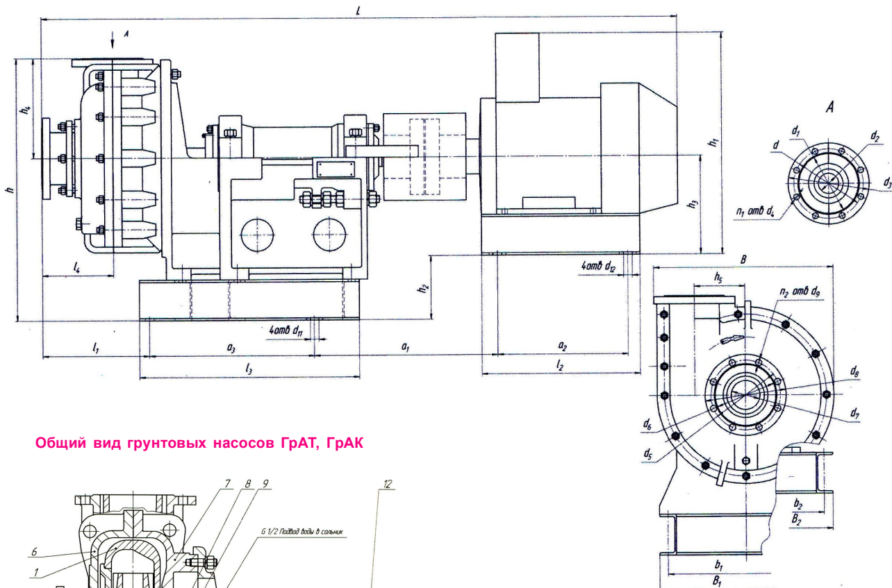
Габаритные и присоединительные размеры насосных агрегатов на базе грунтовых насосов типа ГрАТ (гр. А) СОЕДИНЕНИЕ ЧЕРЕЗ МУФТУ
